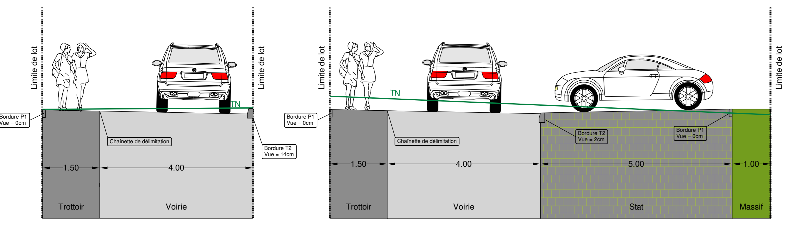
Coupe AA'
